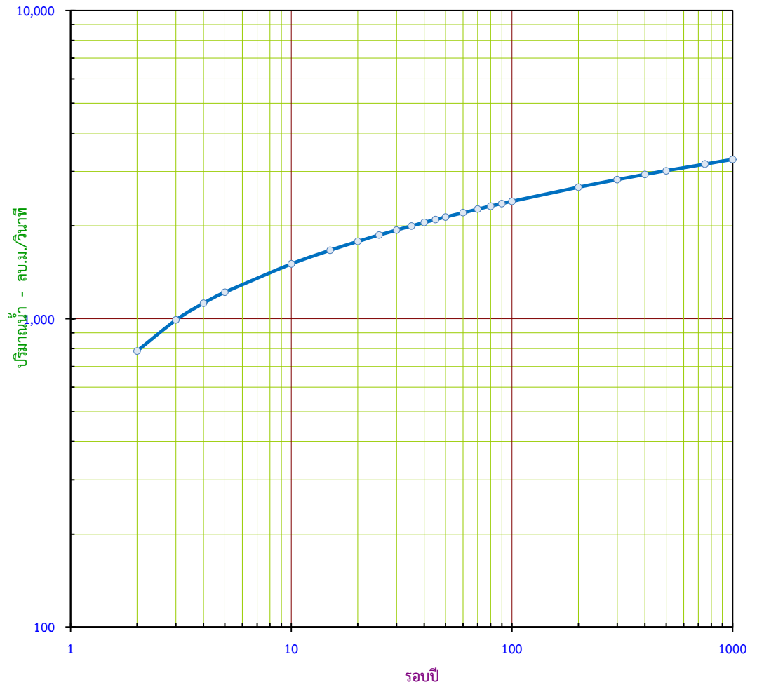
กราฟแสดง ปริมาณน้ำสูงสุดรายปี ขนาดรอบปีต่างๆ สถานี N.12A บ.หาดไร่ อ.ท่าปลา จ.อุตรดิตถ์
